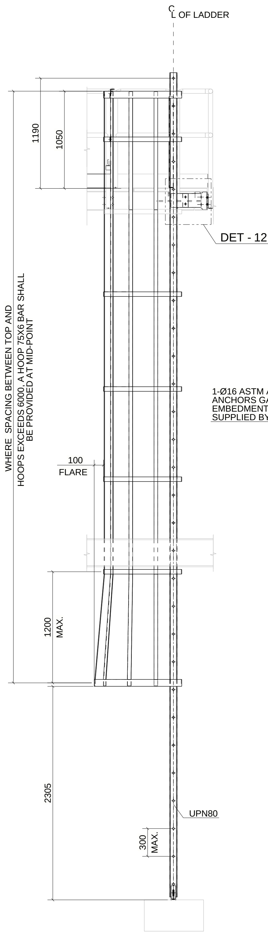
SECTION - 1Q - 1Q
