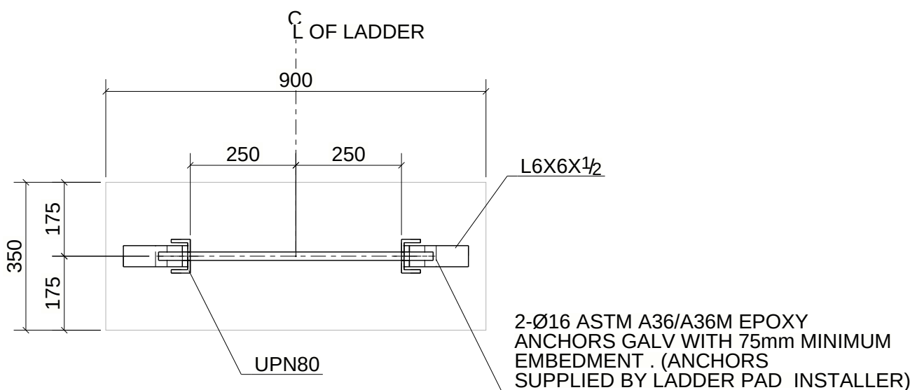
SECTION - 1R - 1R
